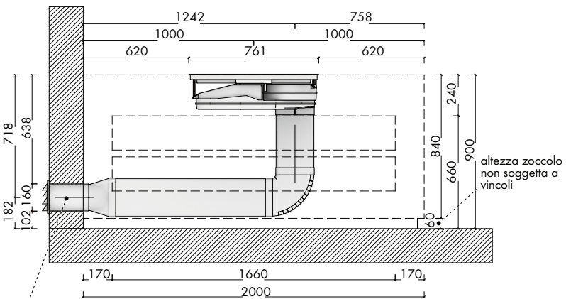
dimensioni foro nella parete per terminale Ø min 160-180 mm; il terminale deve essere ad almeno 20 cm da terra per favorire il deflusso dell'aria
