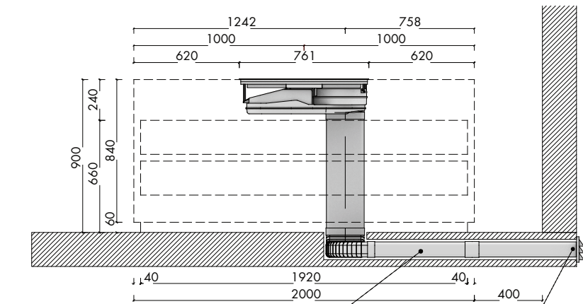
tubazioni nel massetto: prevedere sopra alle tubazioni un rinforzo per compensare i carichi; se le tubazioni usate sono in acciaio non serve il rinforzo dimensioni foro nella parete per terminale min 100x240 mm; il terminale deve essere ad almeno 20 cm da terra per favorire il deflusso dell'aria
